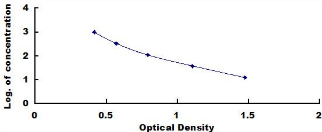
脑啡肽 (ENK) 检测试剂盒标准曲线
